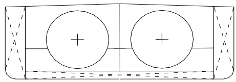
Type C Uitvoering van de ladingtank: 1 Ladingtanktype: 1
